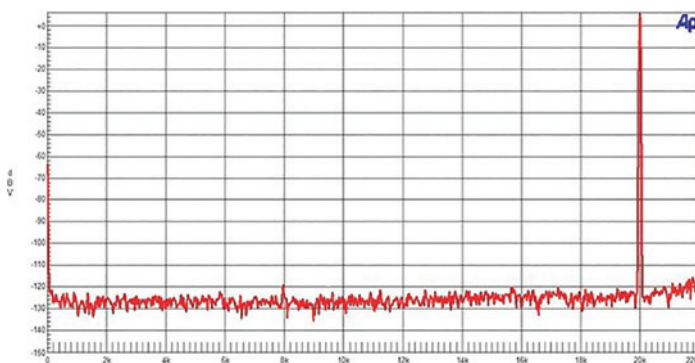
dCS Rossini 20kHz 0dB z dsd
